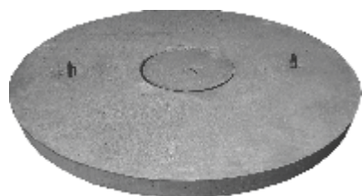
POKROV FI 120/50 Teža: 420 kg kom. na paleti: 5 kom
